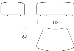
Pouf DO112 112×71×41cm
