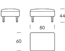
Pouf MA80 80×60×44cm
