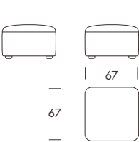
Pouf DO67 67×67×41cm
