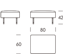
Pouf LM80 80×60×42cm
