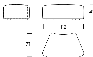
Pouf DO112 112×71×41cm
